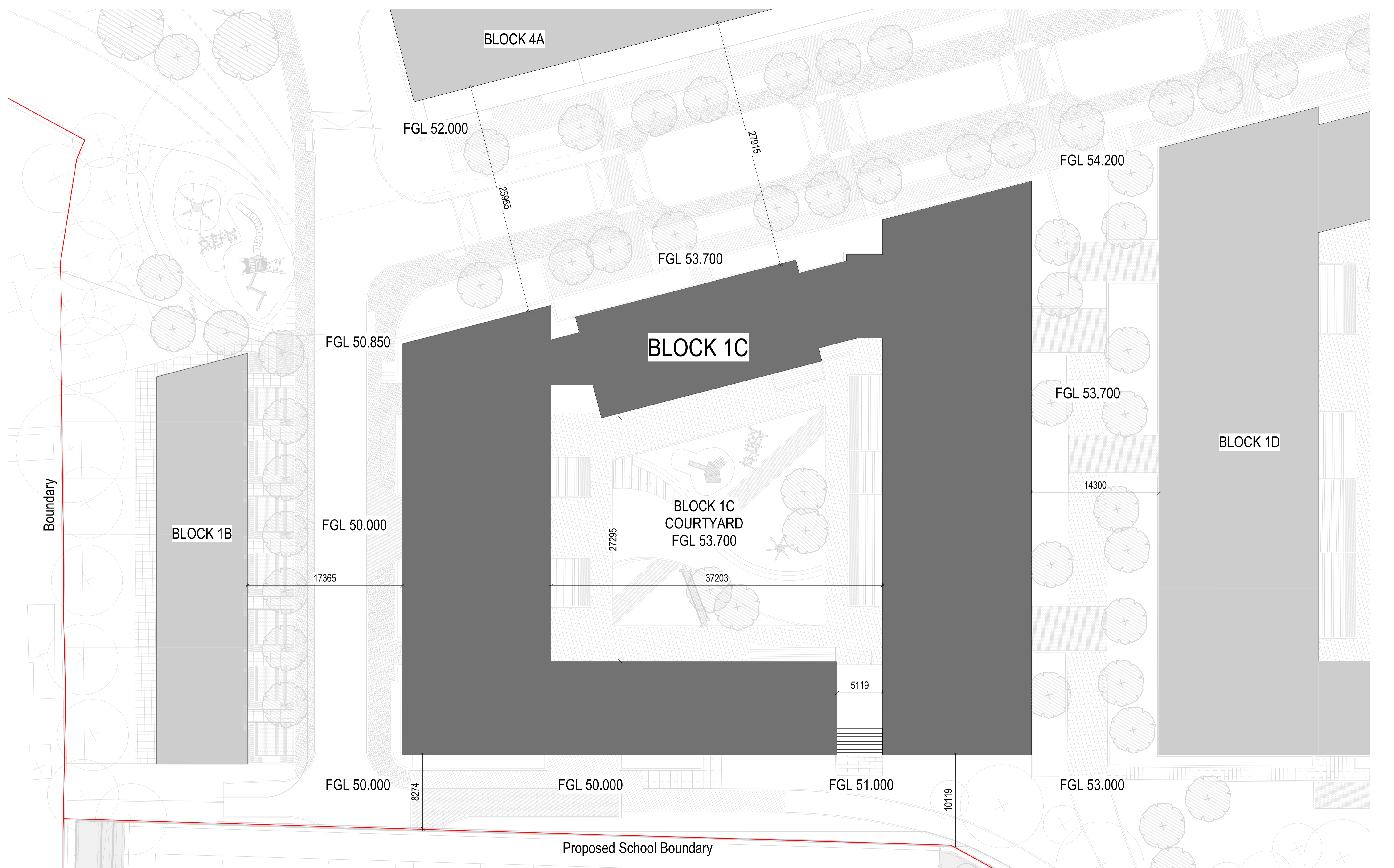
1 Block 1C_Site Plan 1 : 200
