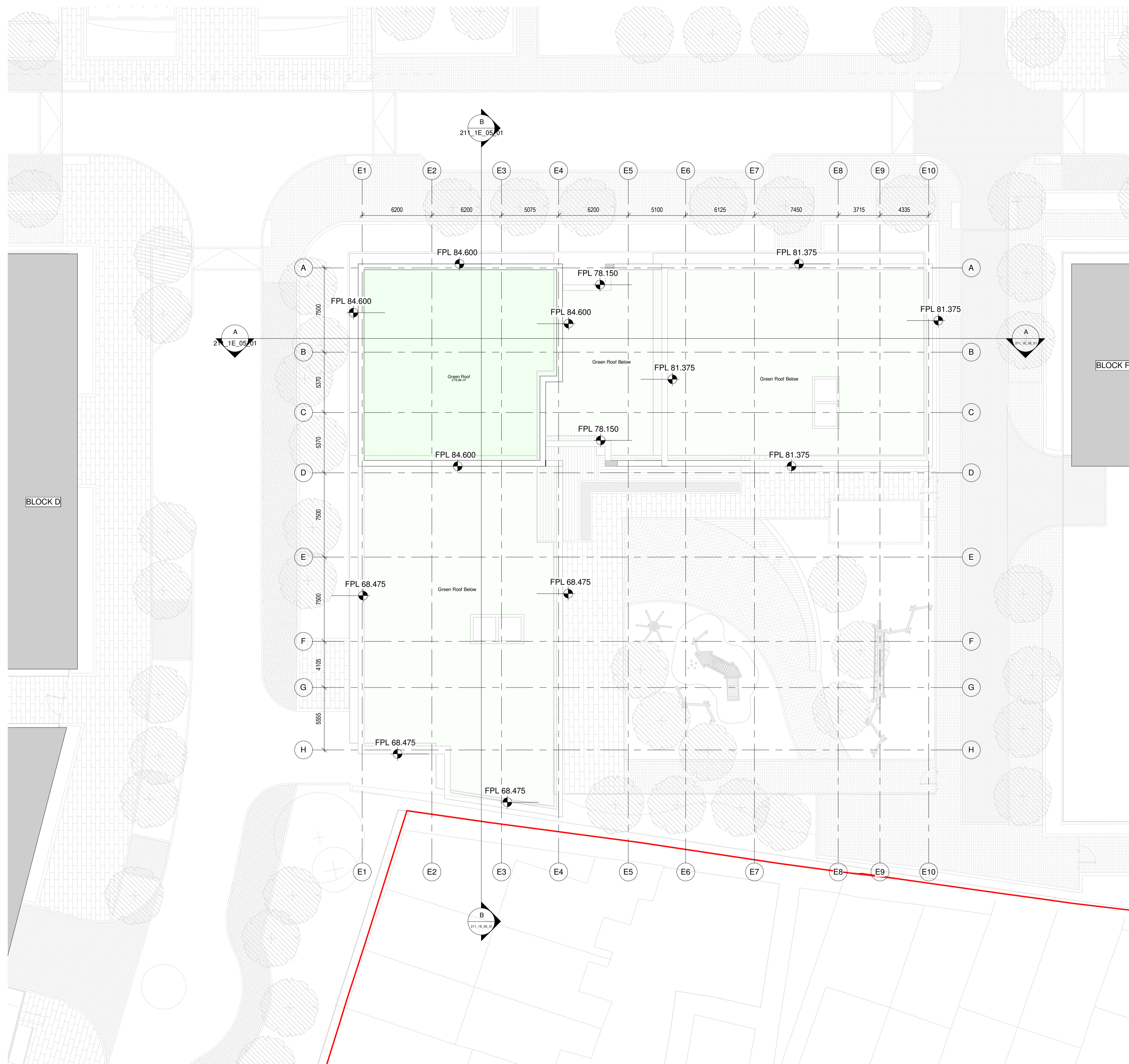
1 Block 1E_Roof Plan 1 : 200
